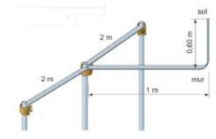
Prise de terre paratonnerre Par piquets alignés
