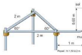
Prise de terre paratonnerre Par piquets triangulés
