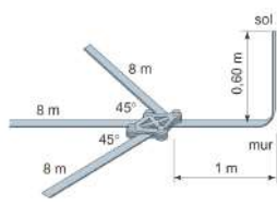
Prise de terre paratonnerre Système patte d'oie
