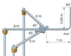
Prise de terre paratonnerre Système patte d'oie améliorée
