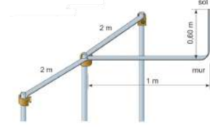
Prise de terre paratonnerre Par piquets alignés
