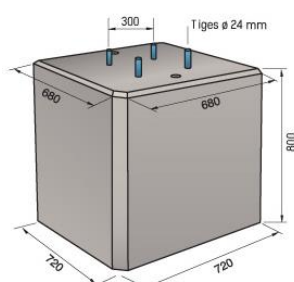
Exemple massifs hors sol Example bases out of the soil Ejemplo masivos fuera del suelo
