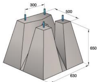
Exemple massif à enterrer Example base to bury Ejemplo masivo a enterrar
