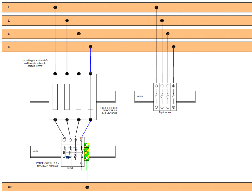
Principe parafoudre Type I installé en armoire TGBT Class I surge protective device principle installed in LVMB Principio supresor de pico tipo I instalado en armario TGBT
