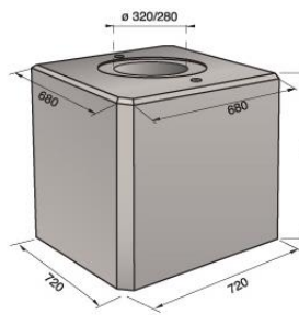
Exemple massifs hors sol Example bases out of the soil Ejemplo masivos fuera del suelo
