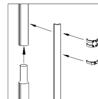
Recubrimiento de los mástiles y fijación del conductor
