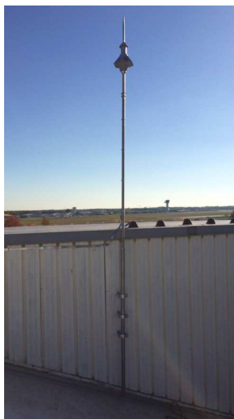
Active ZD ® fixé avec des pattes AFZ0420PD / trépied AFD3300FS et dalles AFH8045DA
