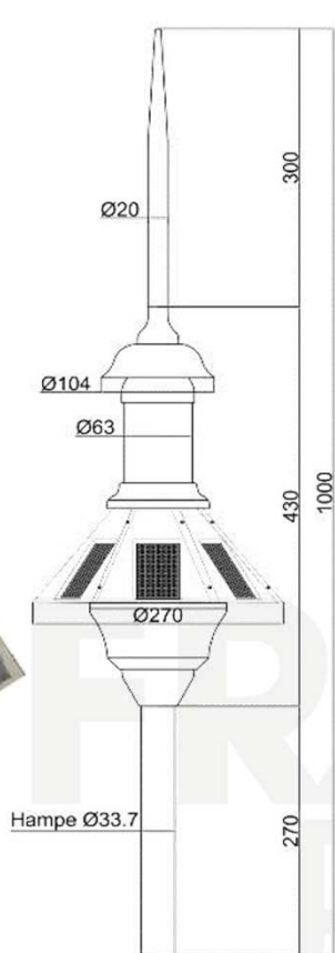
Dimensiones (mm)
