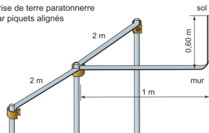
Prise de terre paratonnerre par piquets triangulés
